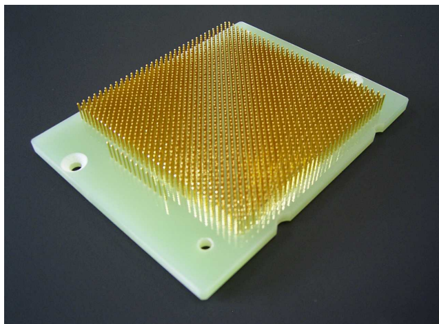
圧入タイプ2048ピン
