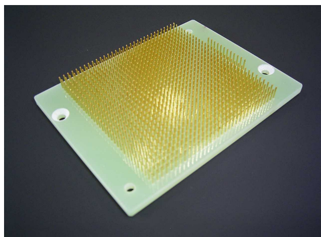
圧入タイプ1024ピン
