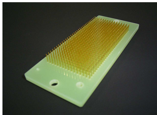
圧入タイプ512ピン
